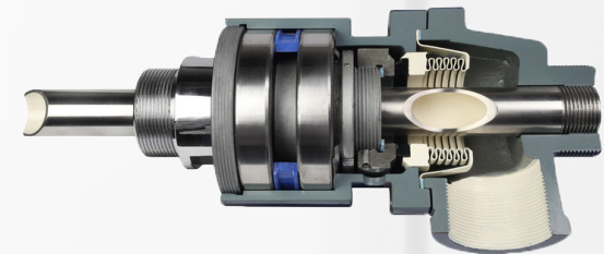
Roterande koppling i genomskärning.
