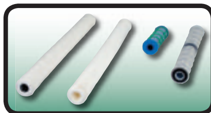
20” lindade filterpatroner för nominell filtrering. Till höger silduksfilter i polymera material men med duk i både polymer alt. Metall. Dessa är standard 10” längd och passar i alla filterhus genom förlängning.
